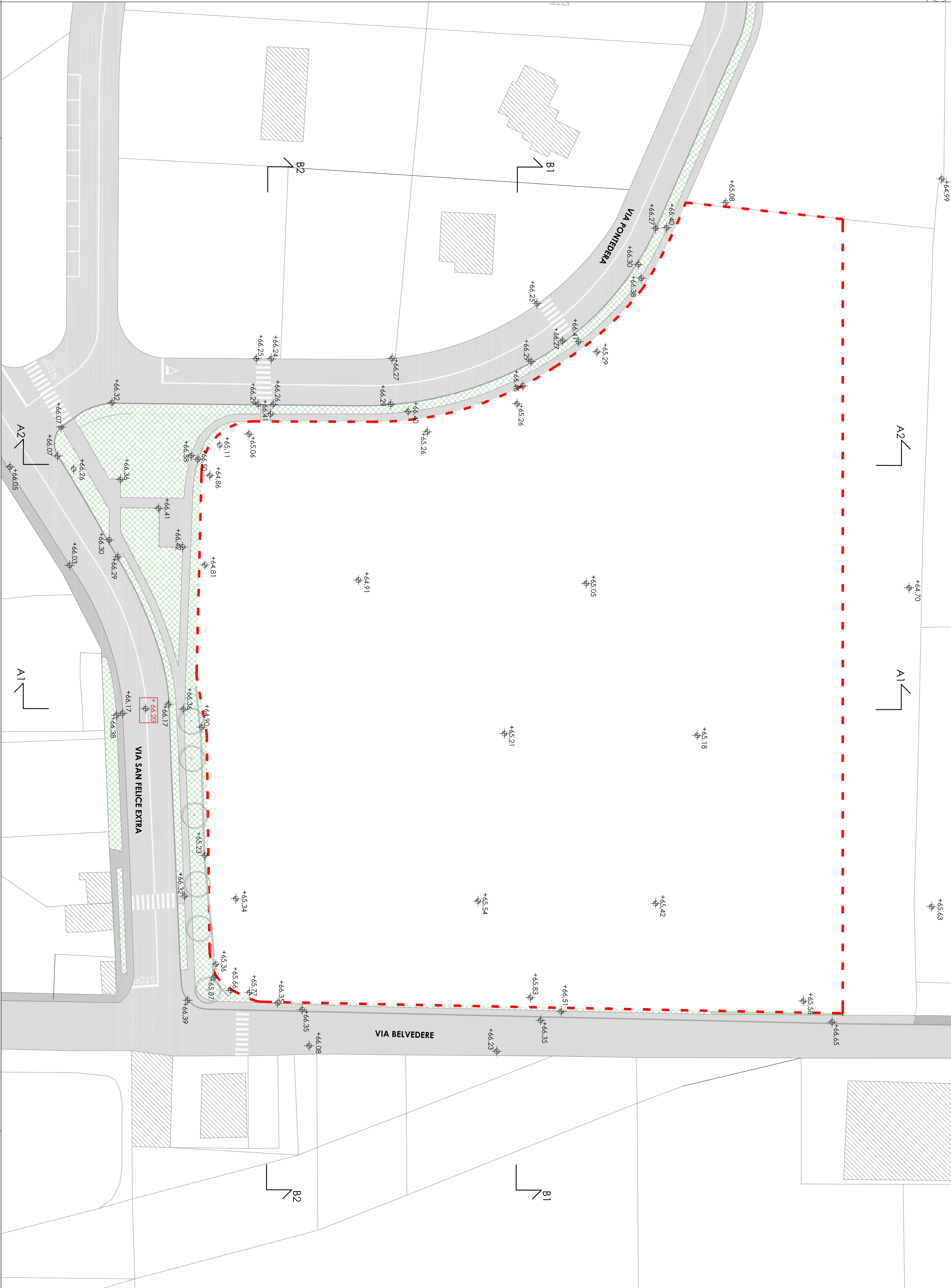
PLANIMETRIA STATO DI FATTO - SC 1:500
